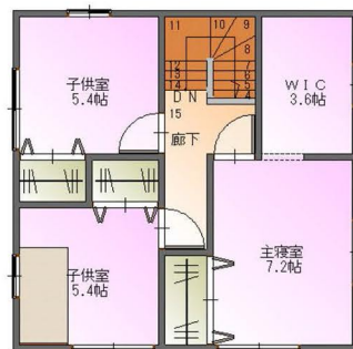
2階平面図
