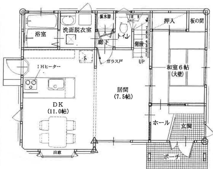
1F平面図
