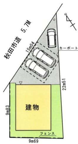
配置図
