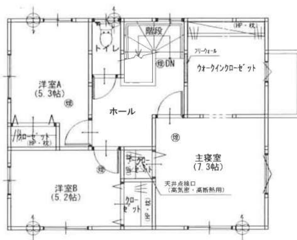
2F平面図
