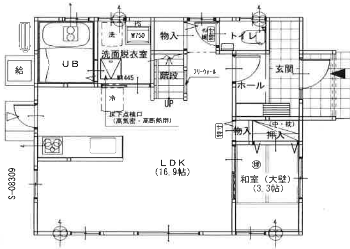
1F平面図
