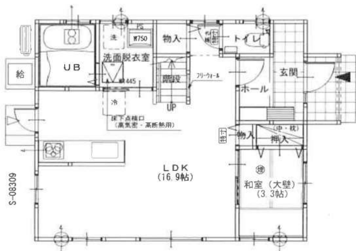
1F平面図
