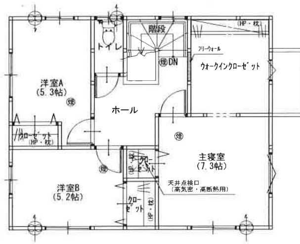
2F平面図
