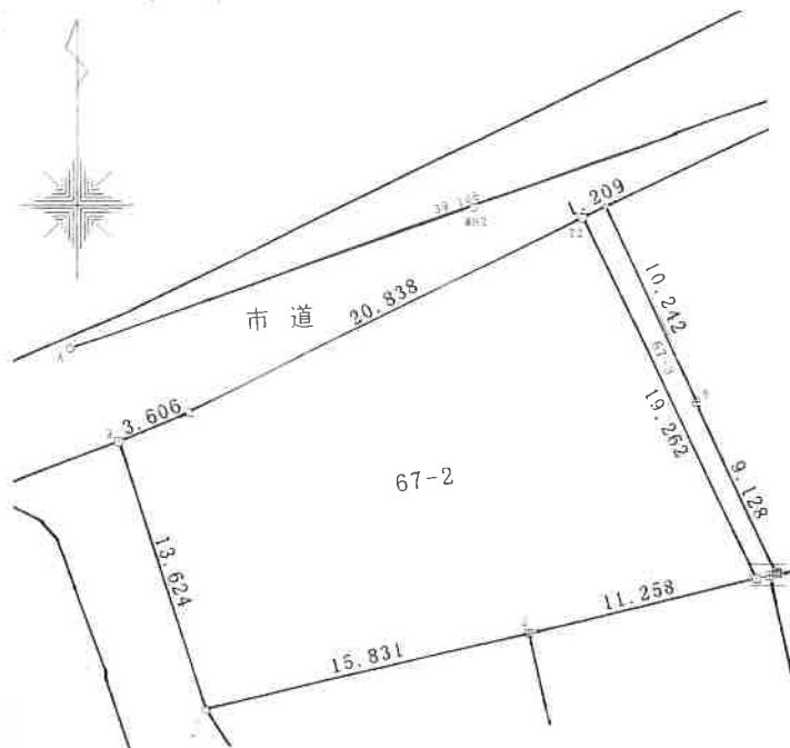
測量図
